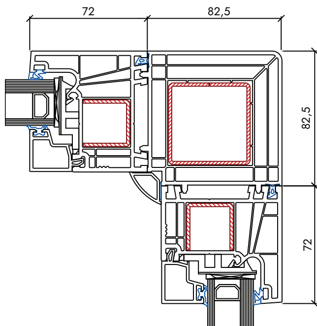
Accoppiamento 90 gradi
