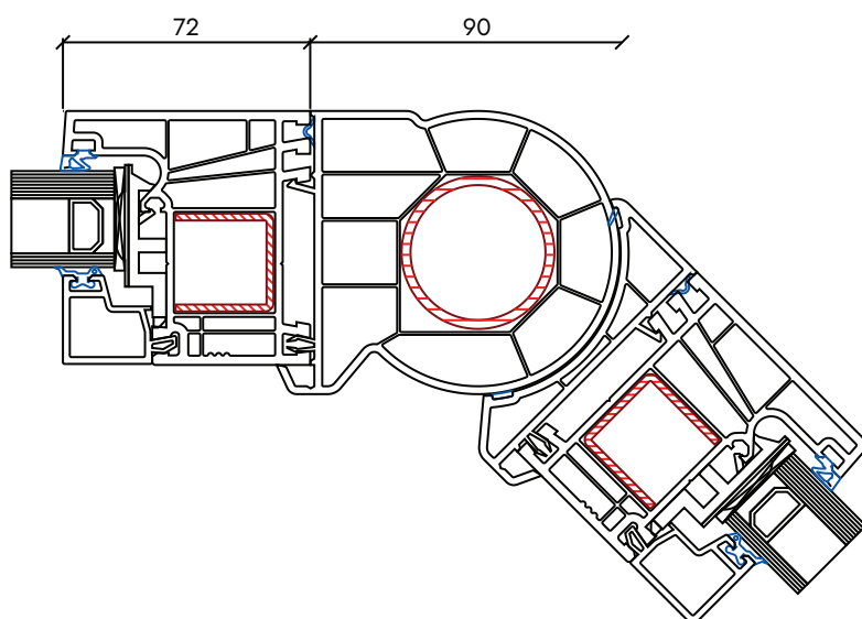
Accoppiamento angolare variabile
