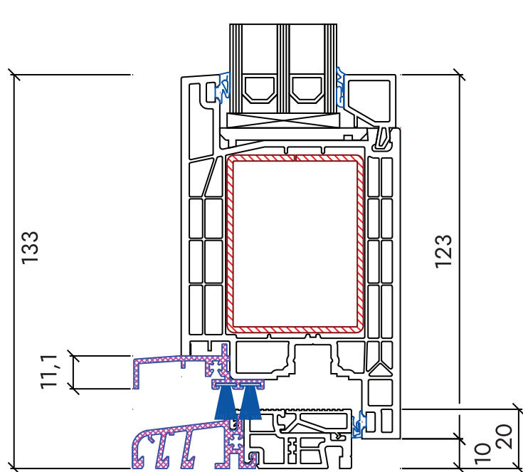
7088 + Soglia Alluminio + Gocciolato Al.
